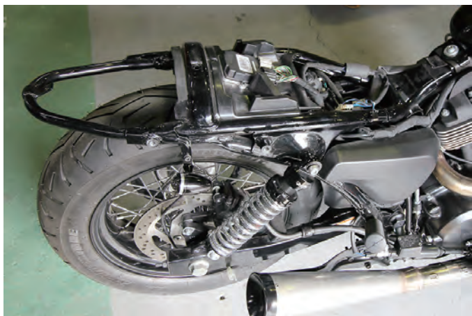
純正シートを取り外します
